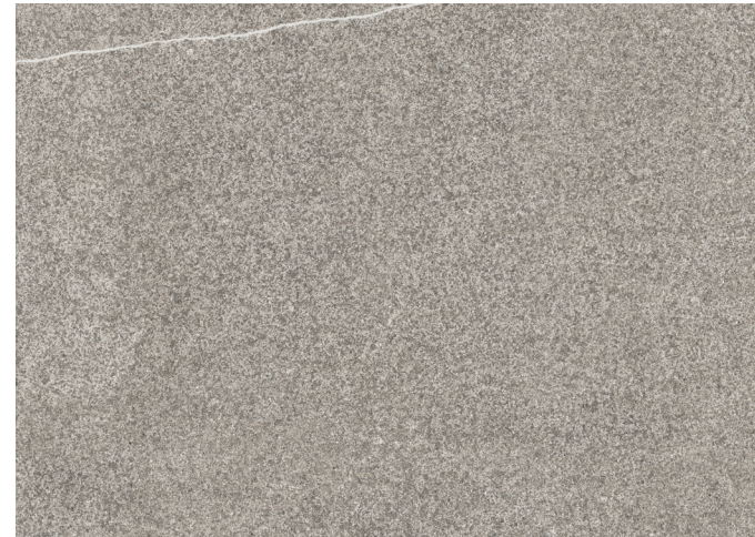
Feldspar
